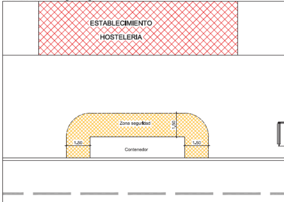
Distancias mínimas de seguridad fig. 3
