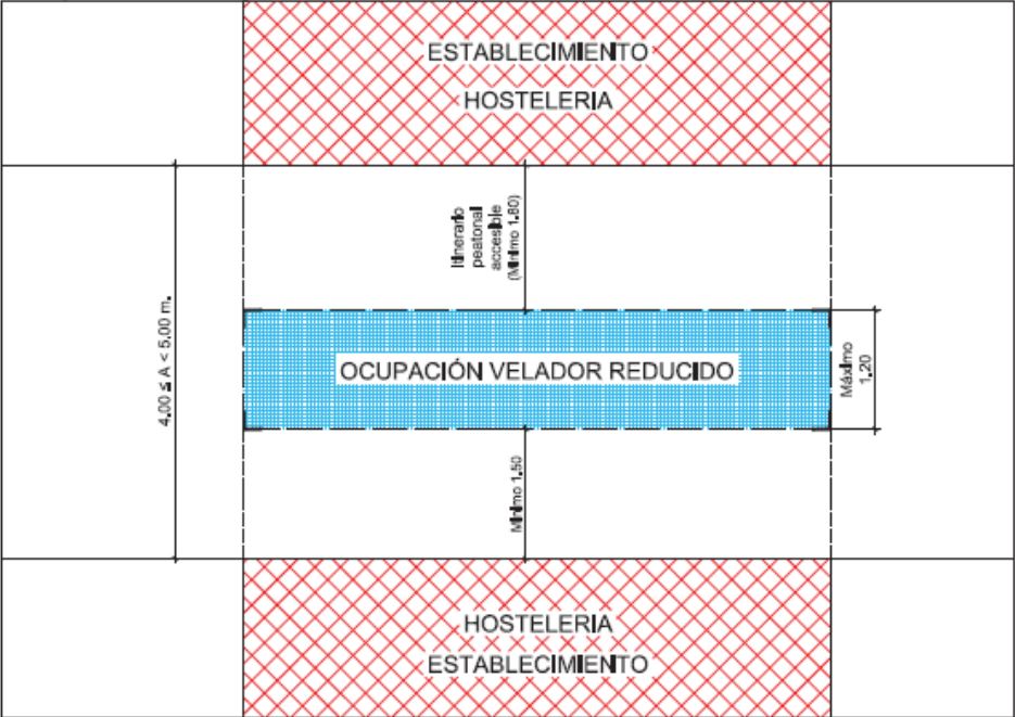
Calles peatonales Aceras fig. 2
