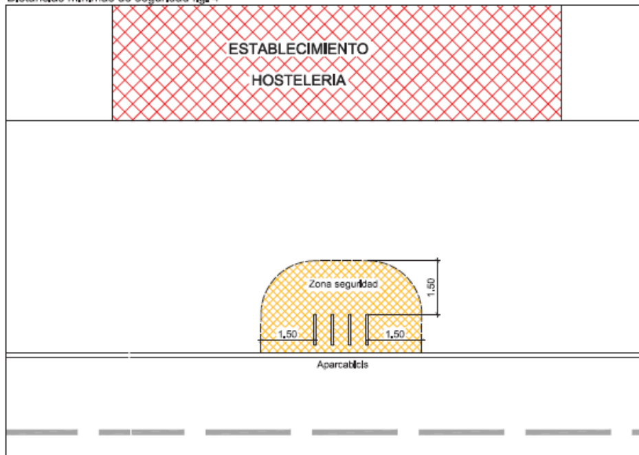
Distancias mínimas de seguridad fig. 4
